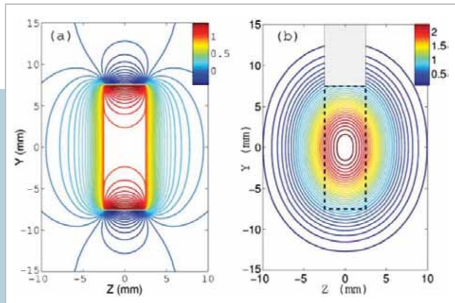
მაგნიტური ველის განაწილება
